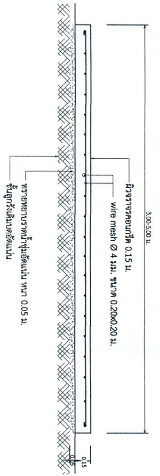
แสดงรูปตัดถนน หน้า 0.15 ม. มาตราส่วน 1 : 25
